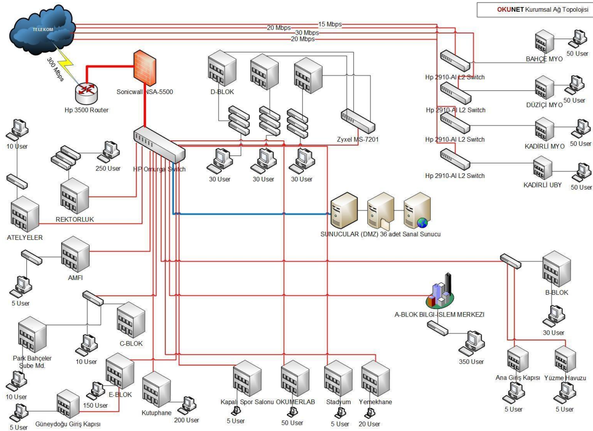
Şekil 2: Osmaniye Korkut Ata Üniversitesi Ağ Planı
